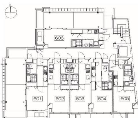
6階平面図
