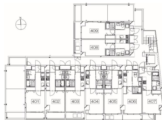
4階平面図
