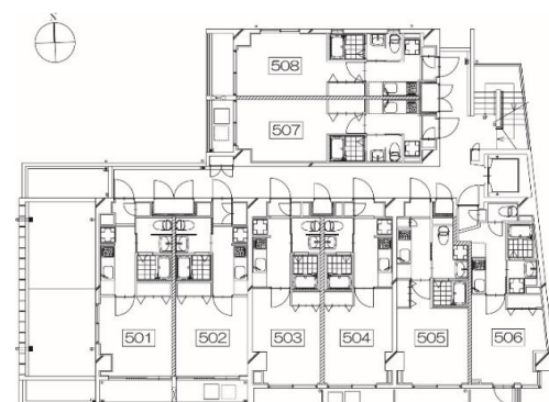
5階平面図
