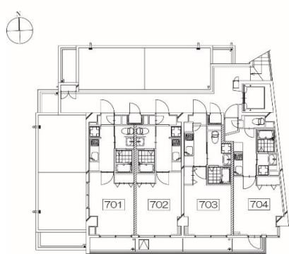
7階平面図
